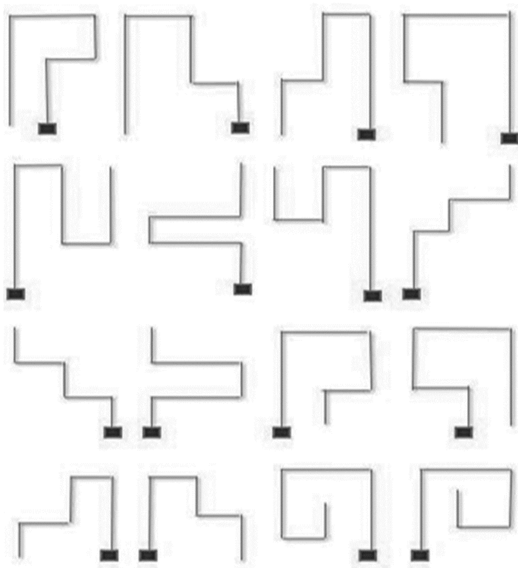
Рисунок 20. Схемы прокладки следового маршрута в FCI IFH-1.
