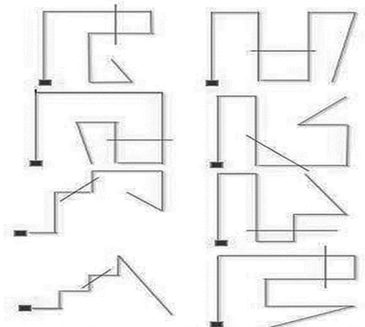
Рисунок 21. Схемы прокладки следового маршрута в FCI IFH-2.
