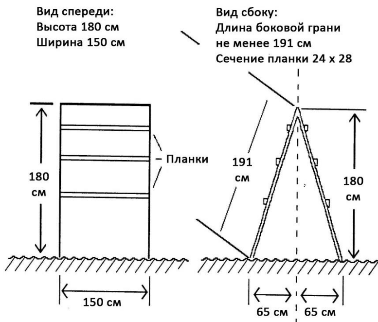
Рисунок 3. Конструкция и параметры наклонной стенки.
