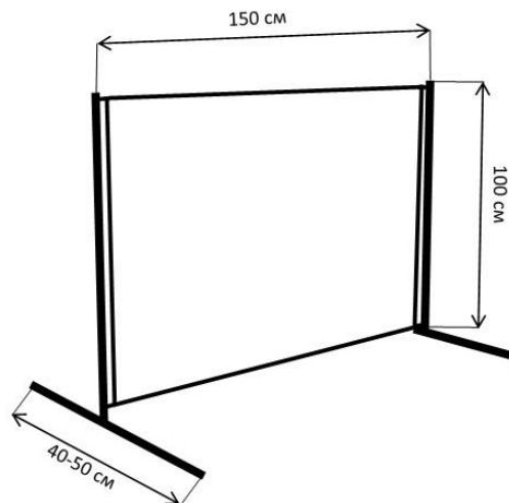
Рисунок 2. Конструкция и параметры барьера.
