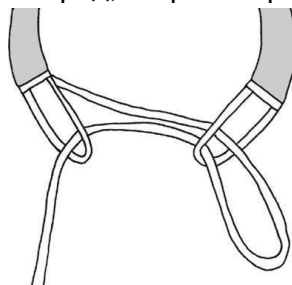
Рисунок 3. Конструкция пускового ошейника
