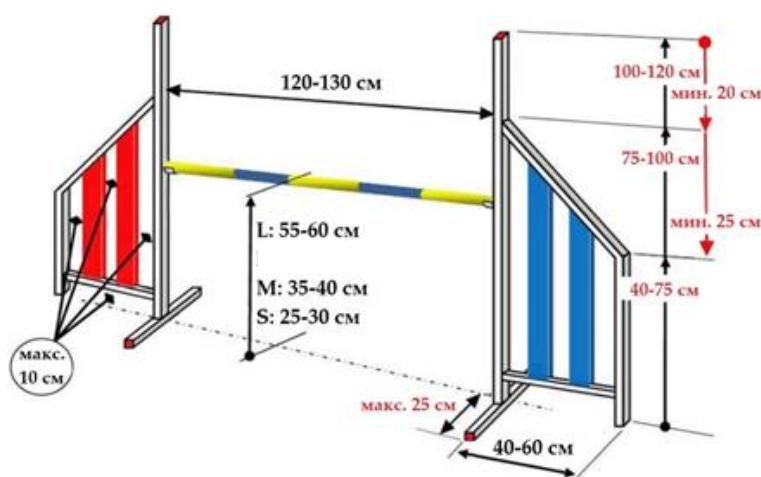
Рисунок 145. Конструкция препятствия «одинарный барьер»
