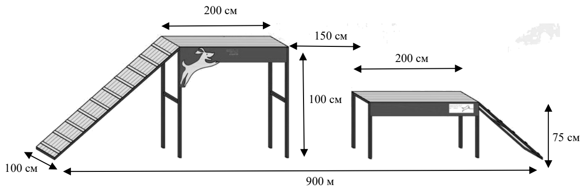
Рисунок 71. Схема препятствия «окоп»
