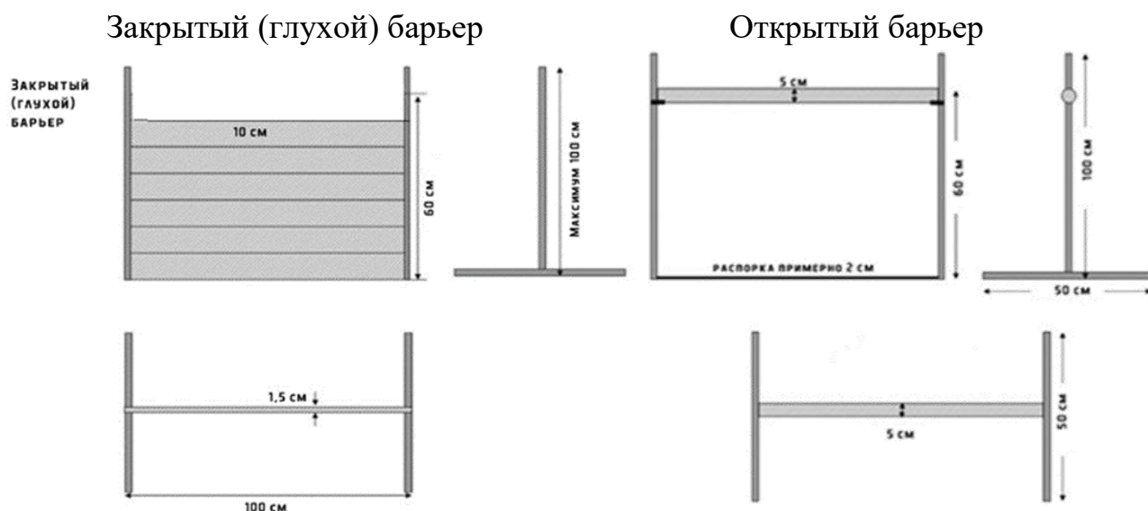
Рисунок 29. Конструкции барьеров
