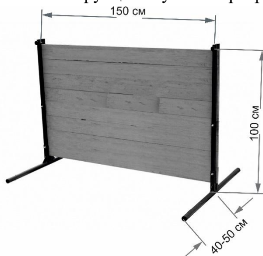
Рисунок 4. Конструкция барьера
