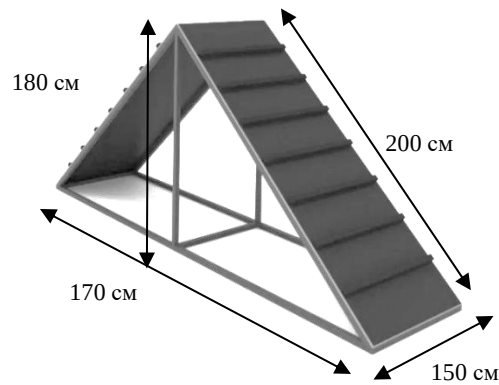
Рисунок 70. Схема препятствия «горка»
