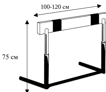
Рисунок 68. Схема препятствия «легкоатлетический барьер»
