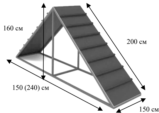
Рисунок 42. Схема препятствия «горка»
