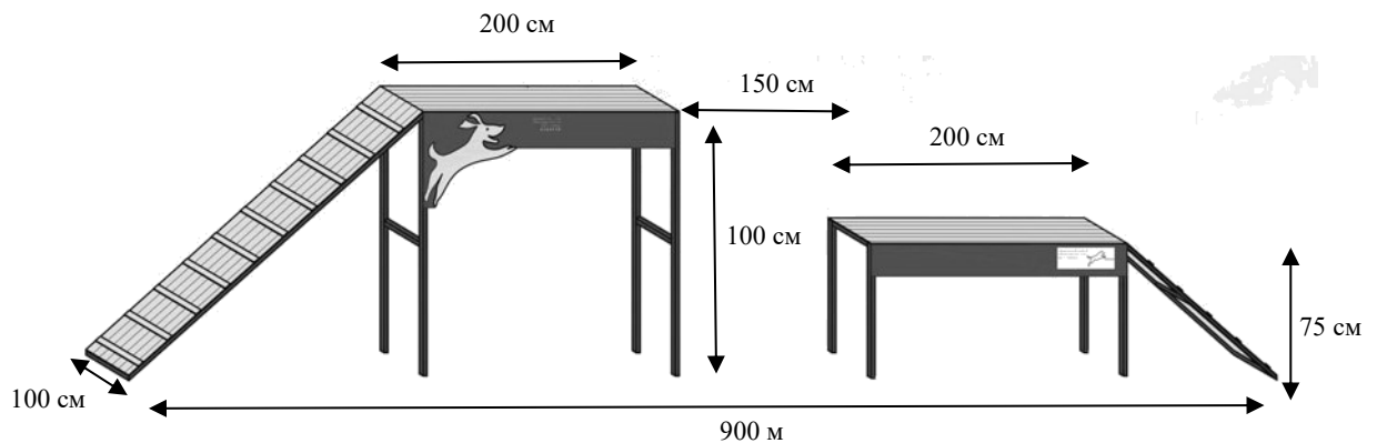
Рисунок 43. Схема препятствия «окоп»
