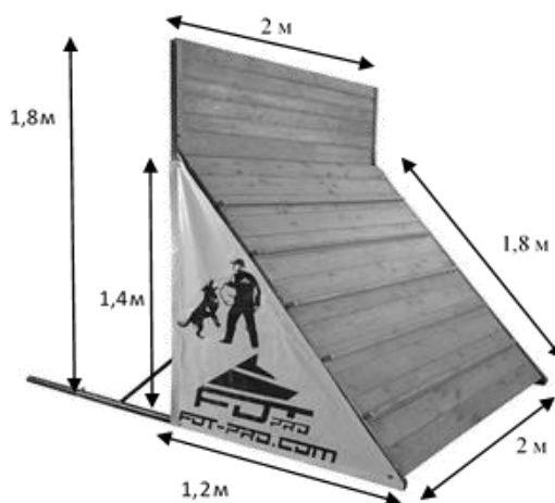
Рисунок 69. Схема препятствия «глухой забор»
