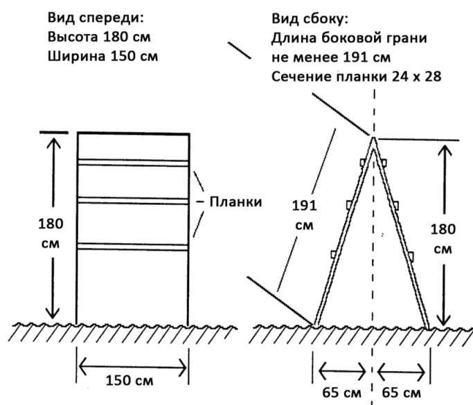
Рисунок 5. Конструкция препятствия «наклонная стенка»
