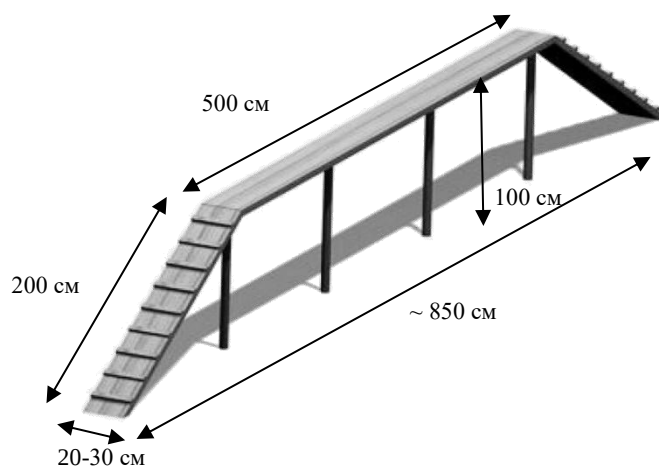
Рисунок 44. Схема препятствия «бум».
