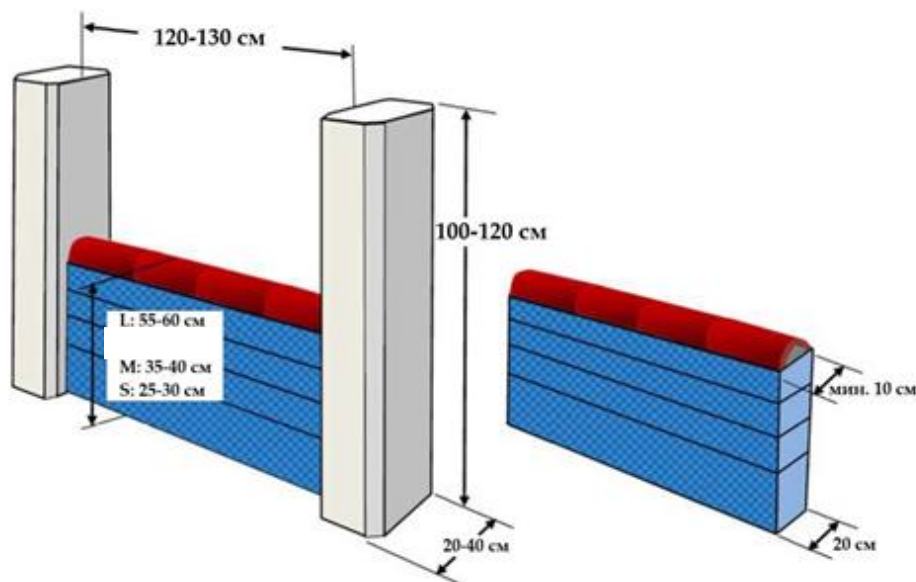
Рисунок 147. Конструкция препятствия «стенка»
