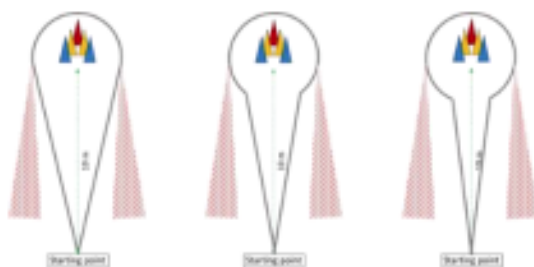
Рис 6. Нормальные траектории обегания конусов
